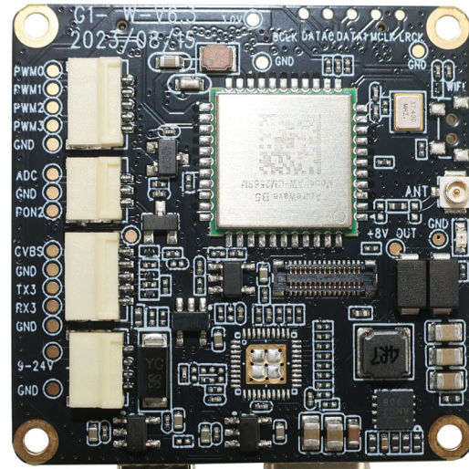
Rückansicht
